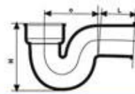
سیفون ۵ درجه
